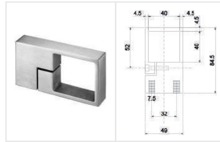
BRK 3055 Conector de estructura metálica a barandal cuadrado tipo abrazadera, para tubo milimétrico. • Material: Acero inoxidable. • Acabado: Satín.
