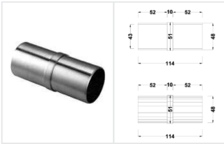
BRK 3054 Conector tubo-tubo recto, para tubo de 2". • Material: Acero inoxidable. • Acabado: Satín.
