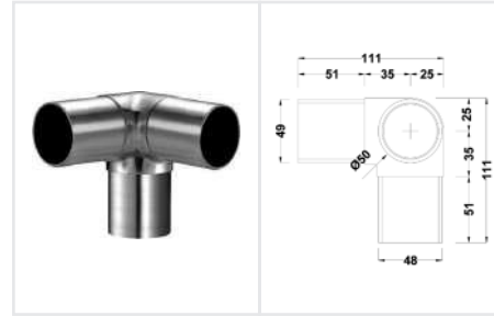
BRK 3053 Conector esquinero 90° en "T" tubo-tubo, para tubo de 2". • Material: Acero inoxidable. • Acabado: Satín.
