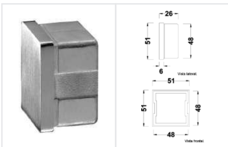
BRK 3058 Tapón para terminación de barandal cuadrado de 2". • Material: Acero inoxidable. • Acabado: Satín.
