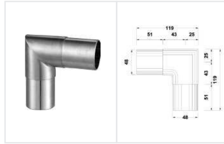
BRK 3051-2 Conector tubo-tubo de 90°, para tubo de 2", esquina angular. • Material: Acero inoxidable. • Acabado: Satín.
