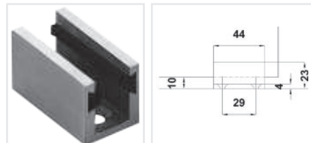
BRK 3850-1D: Guía de piso para kit de baño.
