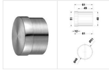
BRK 3057 Tapón para terminación de barandal redondo, para tubo de 2". • Material: Acero inoxidable. • Acabado: Satín.
