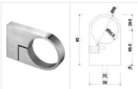
BRK 3056 Conector de estructura metálica a barandal redondo tipo abrazadera, para tubo milimétrico. • Material: Acero inoxidable. • Acabado: Satín.
