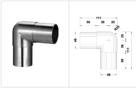
BRK 3051-1 Conector tubo-tubo de 90°, para tubo de 2", esquina redonda. • Material: Acero inoxidable. • Acabado: Satín.
