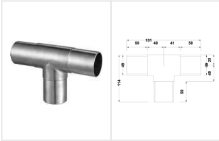
BRK 3052 Conector "T" tubo-tubo, para tubo de 2". • Material: Acero inoxidable. • Acabado: Satín.
