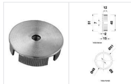
BRK 3059 Tapón plano de poste para barandal redondo para recibir conector de rosca, para tubo de 2". • Material: Acero inoxidable. • Acabado: Satín.
