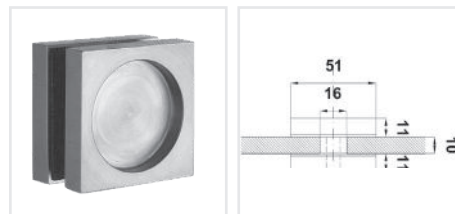
BRK 3850-1H: Manija cuadrada ahuecada de 50 x 50 mm.
